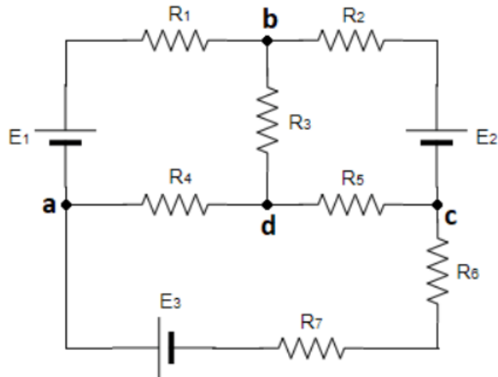
Figura 1. Ejemplo 1 de circuito diagramable por nuestro lenguaje, con paralelos, resistencias, conectores y fuentes.
